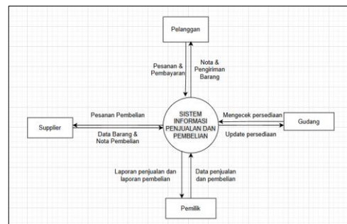
Gambar 2. Diagram Konteks
